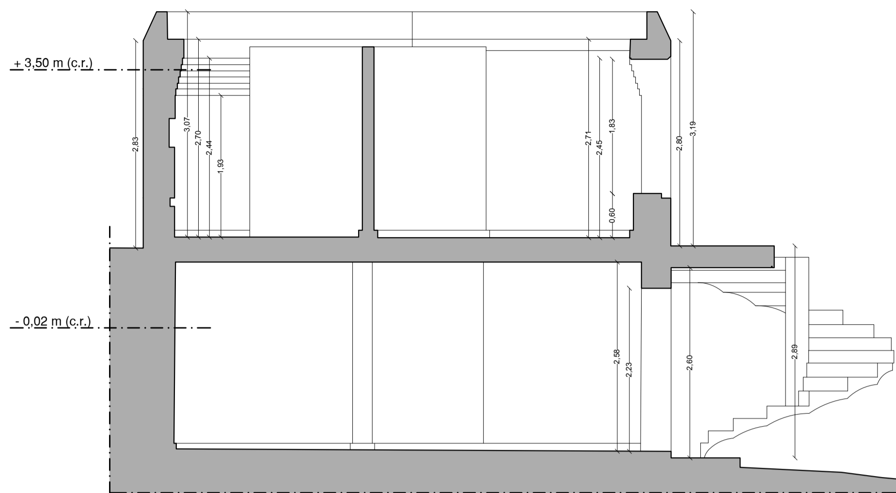
Sección A-A'
