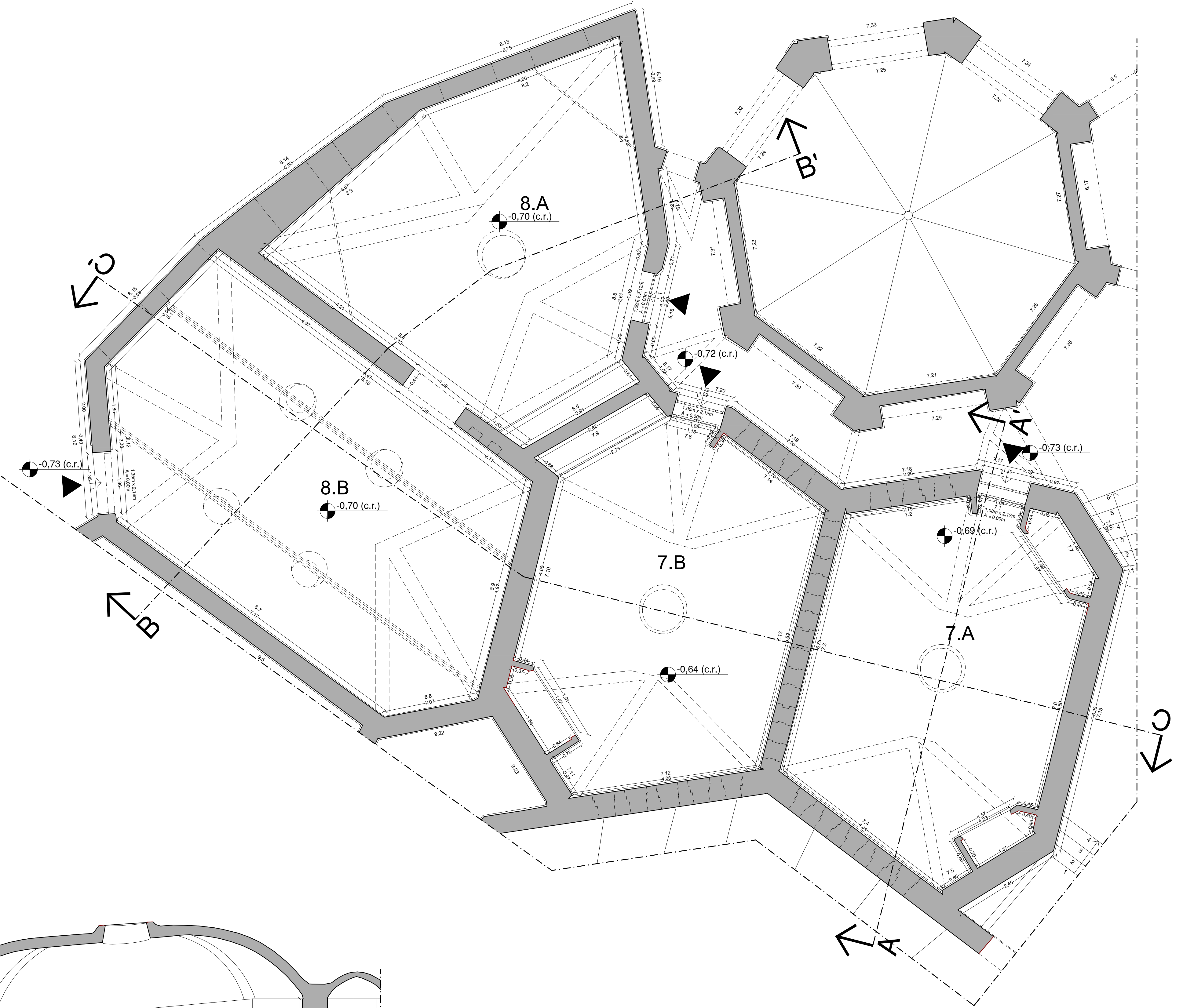
Planta a cota -0,02 (c.r.)
