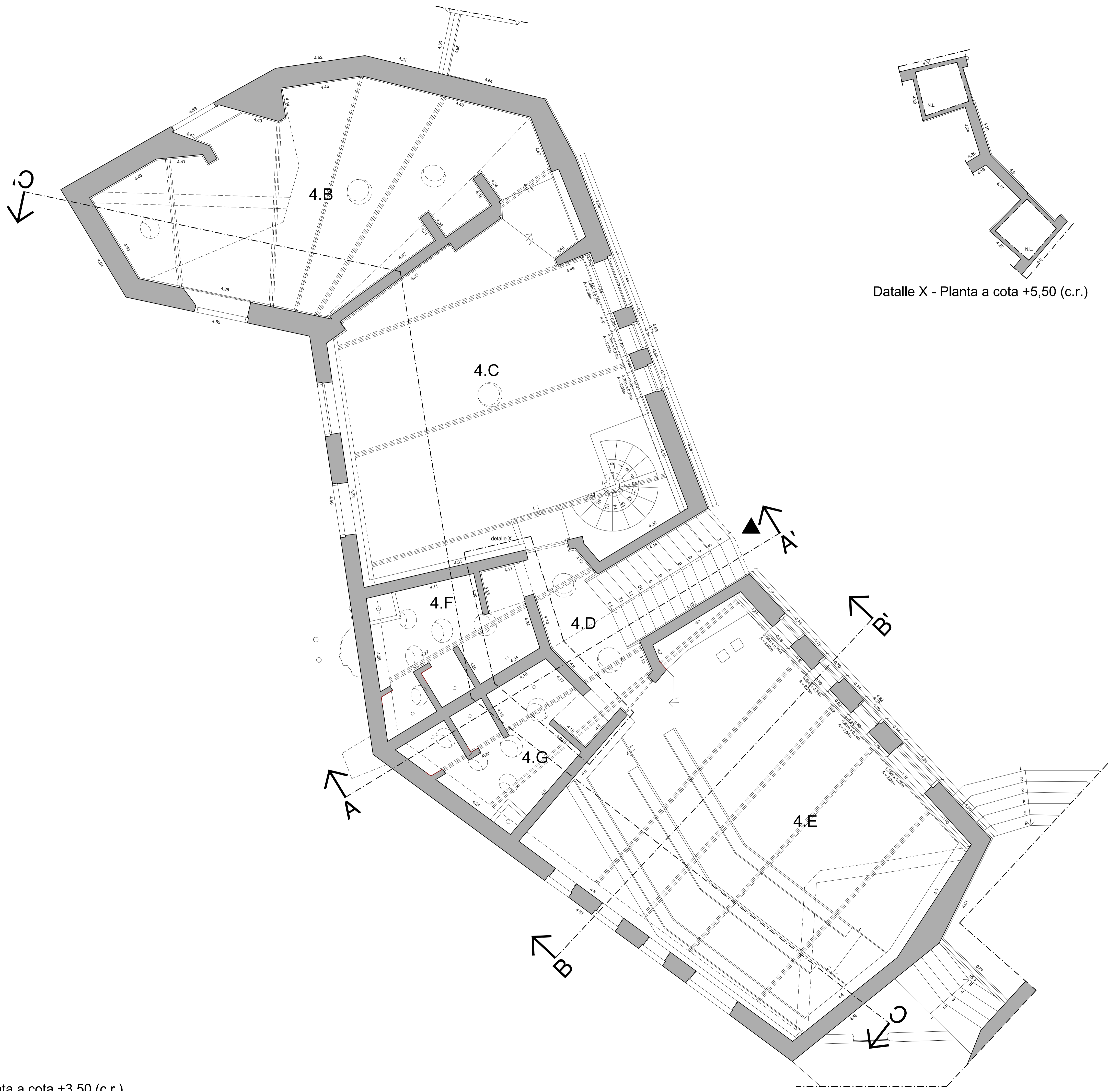
Planta a cota +3,50 (c.r.)
