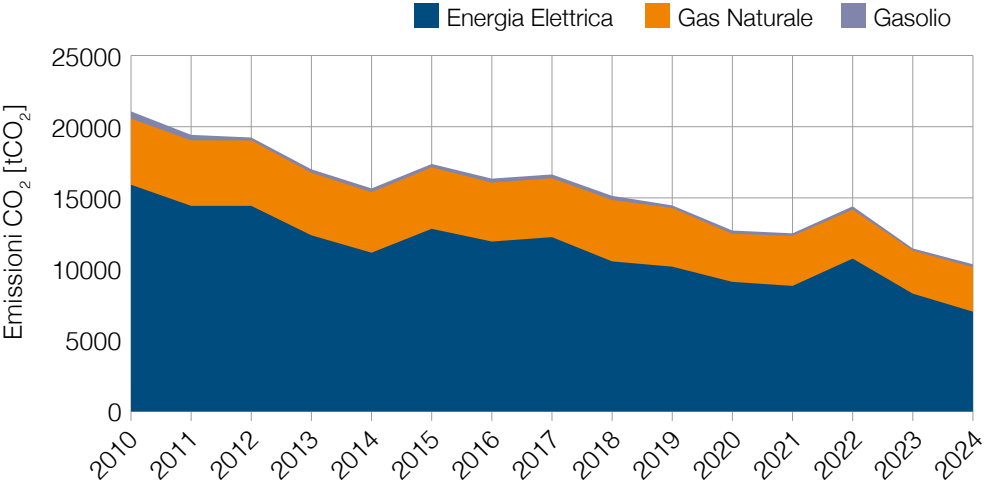
Figura 44 – Storico emissioni CO 2 di Ateneo. Fonte: Energy Manager.
