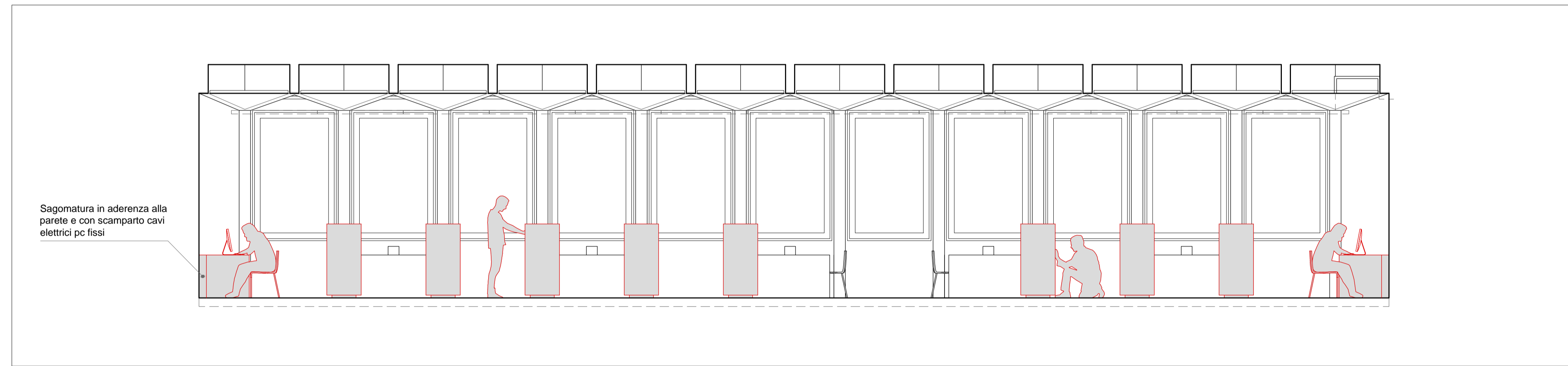
Sezione BB' - Scala 1:50
