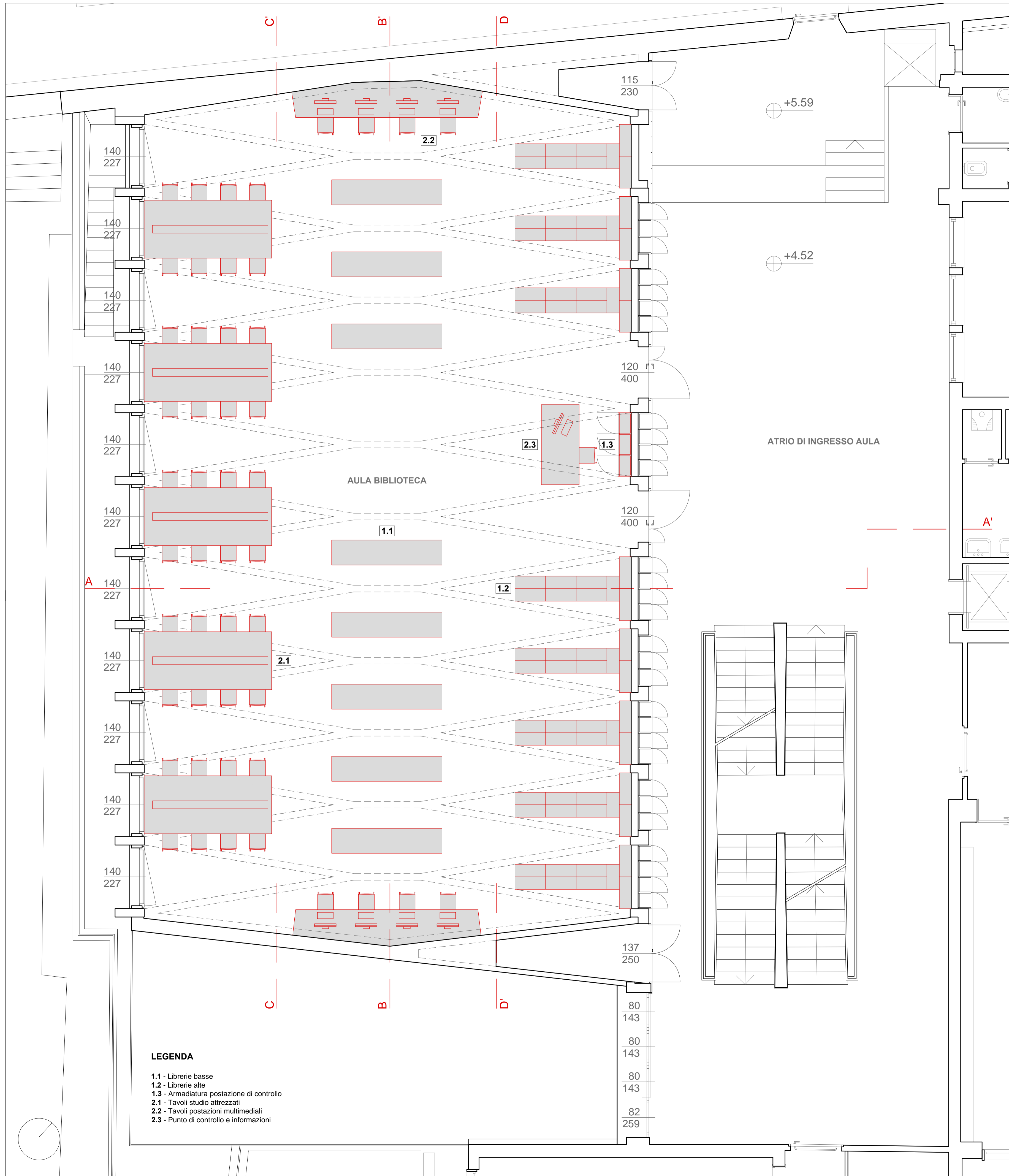
Pianta - Scala 1:50
